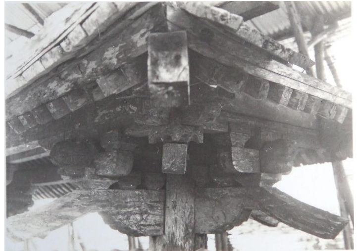
写真 13 上層屋根の隅木。
