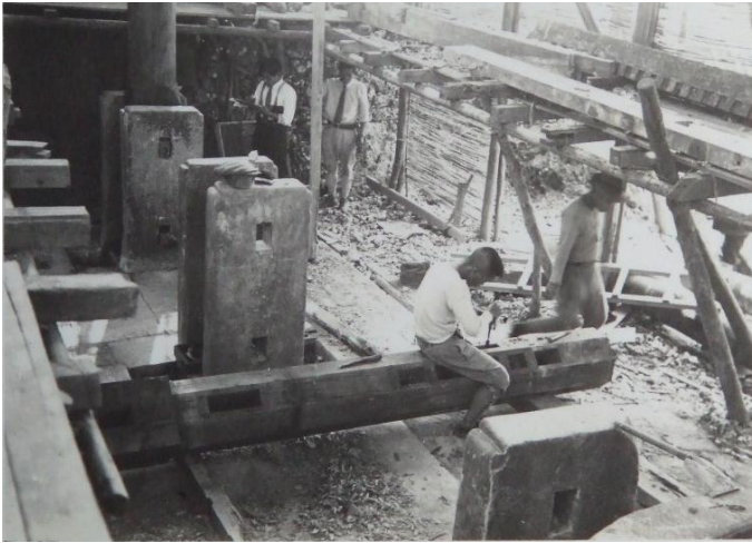
写真6 柱のほぞを加工している。
