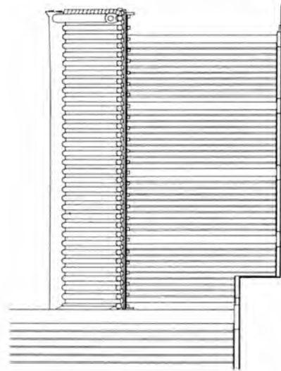
東之廊下 (東側) 1/50
