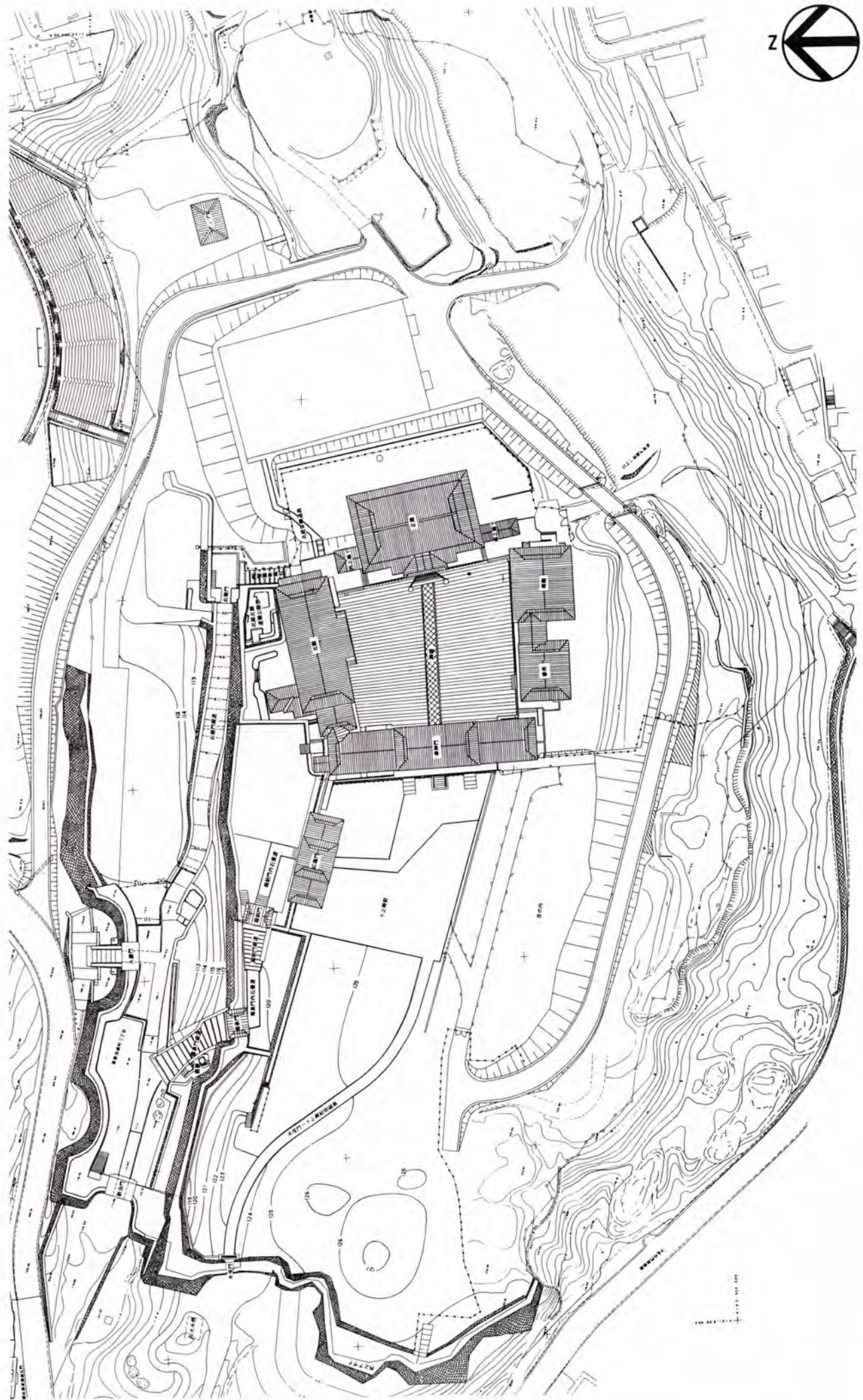
国営沖繩記念公園首里地区 全体配置図
