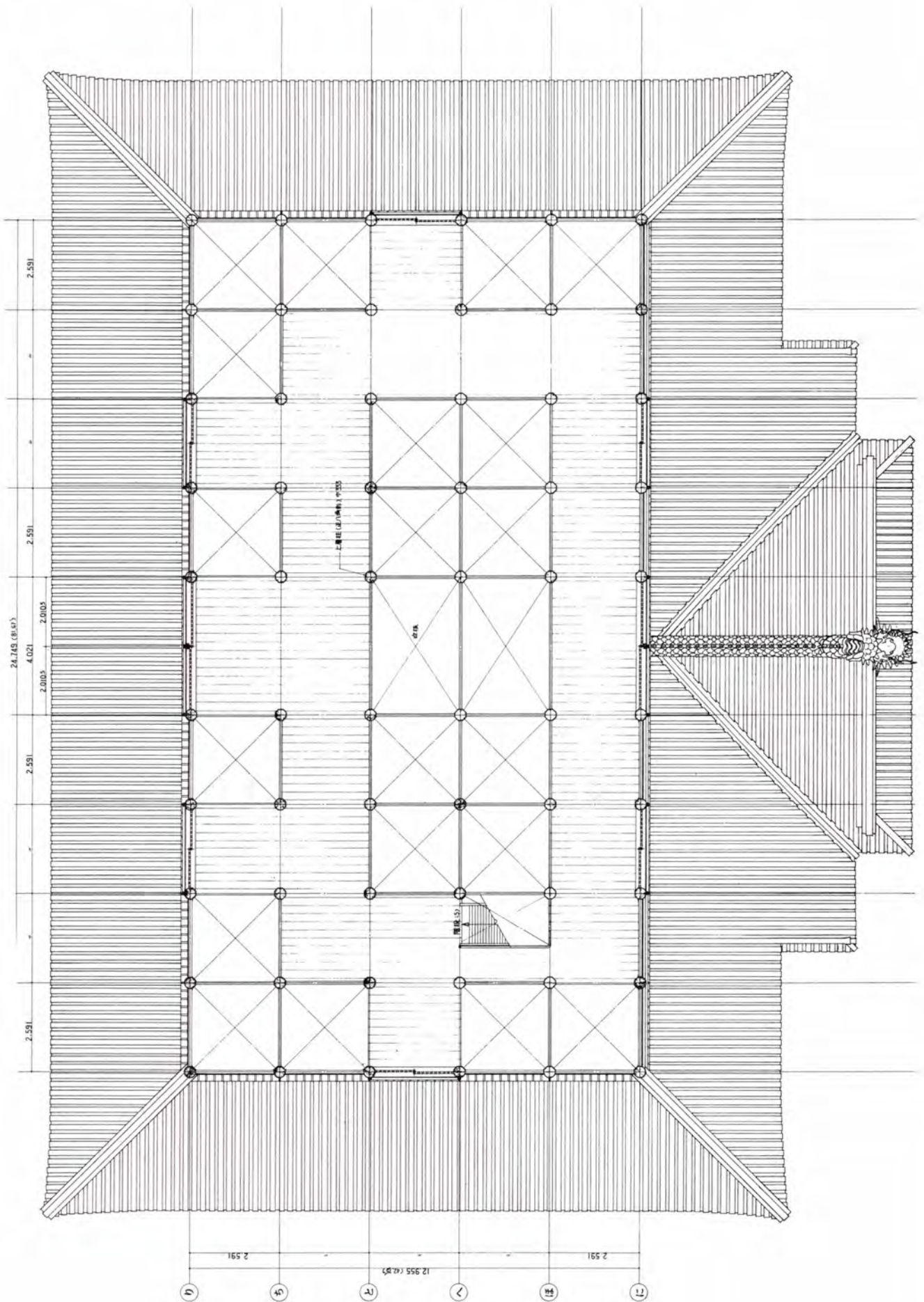
3 樓平面圖 1/50
