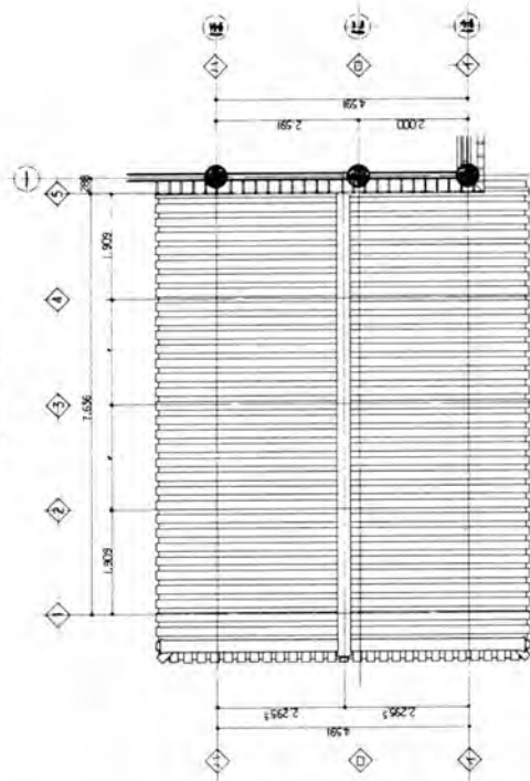
西之廊下 1/50
